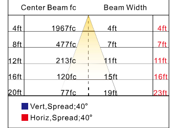
200W/40D
